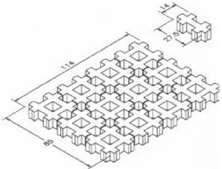
VISTA ISOMETRICA
